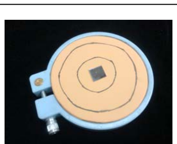
圖 7-3：將 B 圓的圓周記號調整至繃框內框邊緣處，即屬「中度緊繃」。
