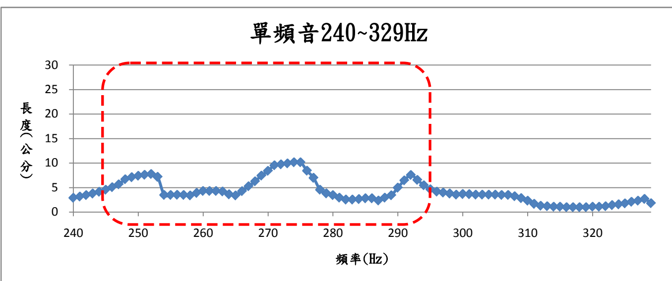
圖 4-3：單頻音介於 240~329Hz 間時，不同的單頻音與其雷射光反射的紅點圖形長度之關係圖
