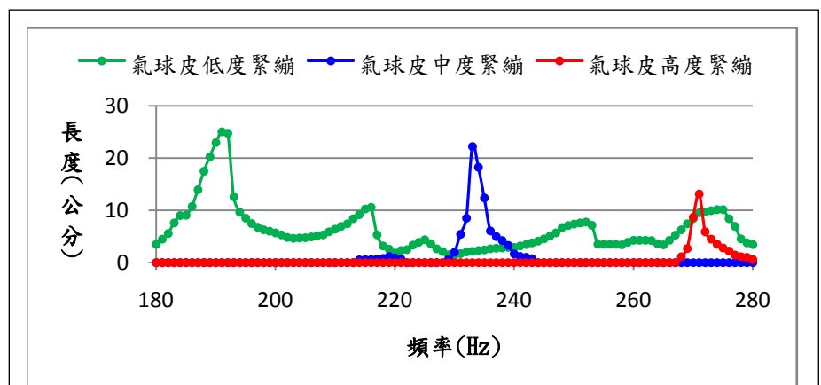
圖 9-11：不同緊繃程度氣球皮能使雷射光筆反射出最大圖形的頻率範圍及其圖形長度關係圖
